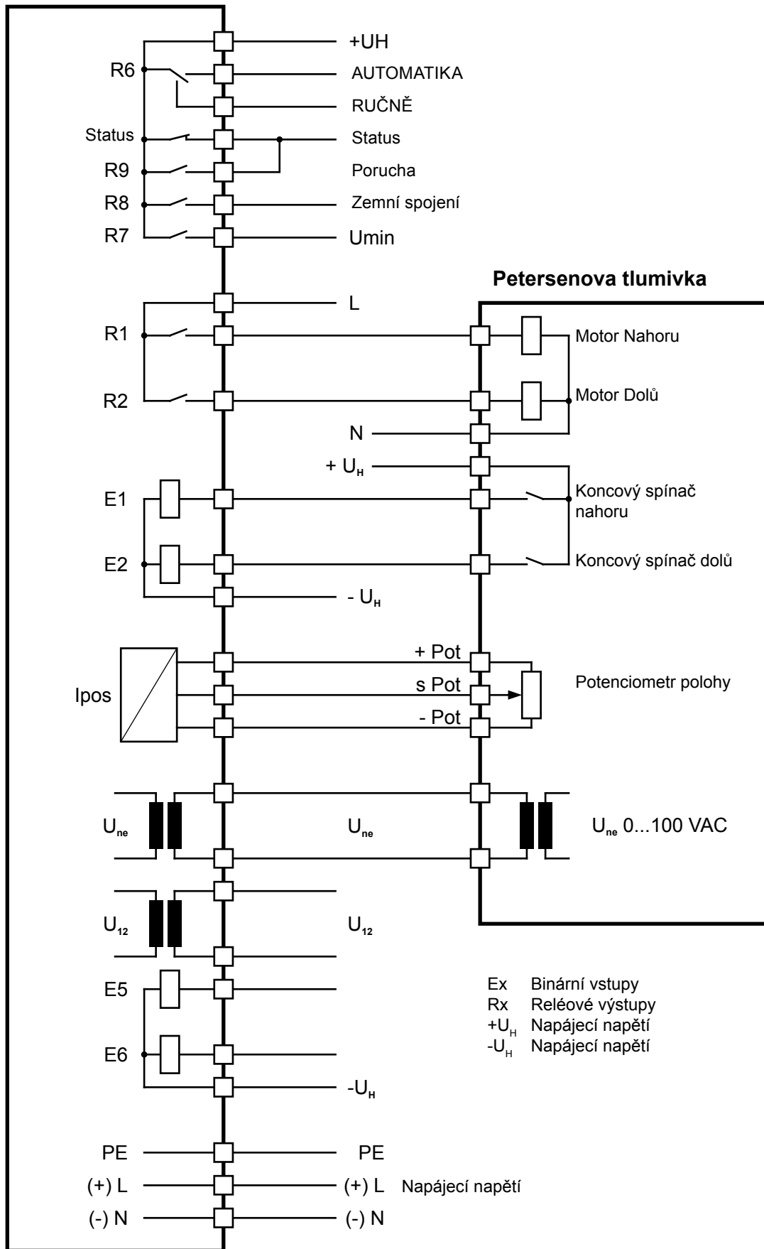
Připojení REG-DP k Petersenově tlumivce
